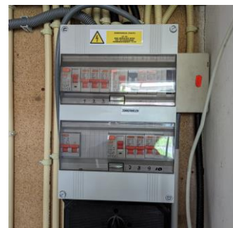
Foto 7: Groepenkast
