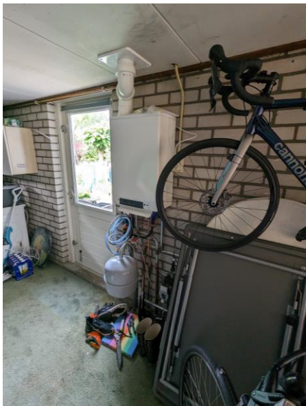
Foto 1: Plek Cv-ketel
