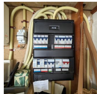
Foto 6: Groepenkast
